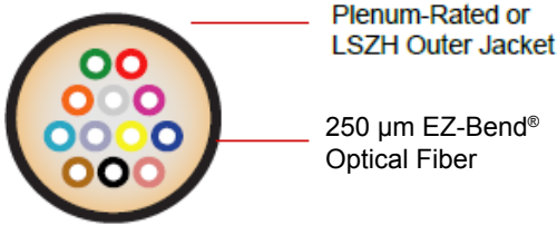
12-Fiber Cable
